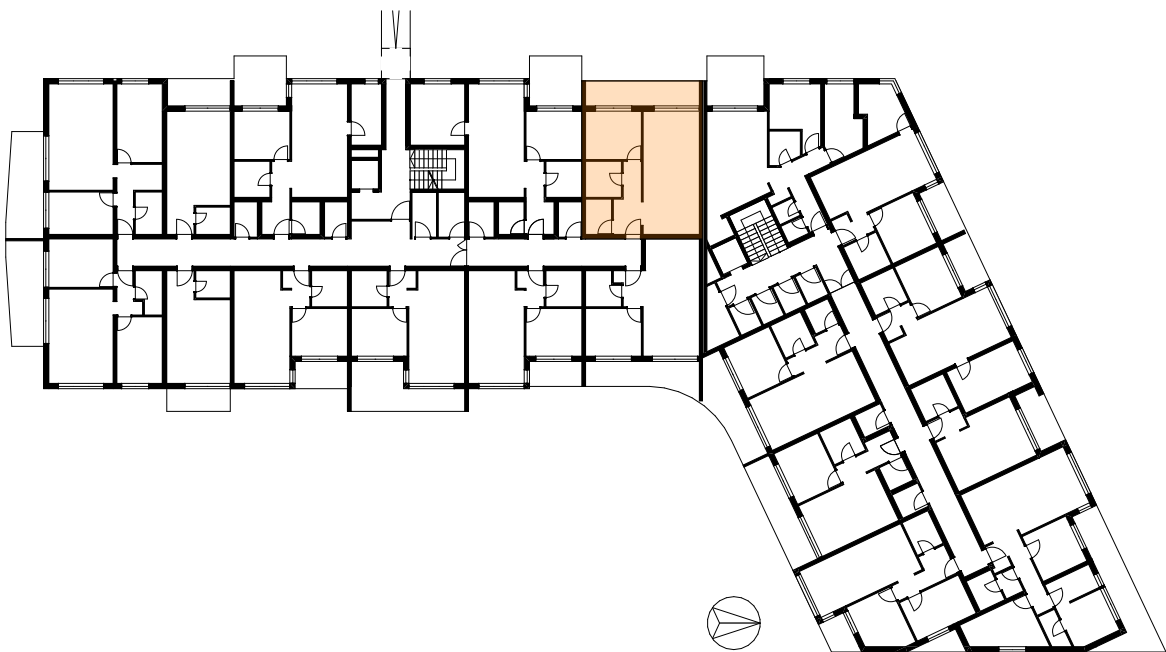
TLOCRT - 2.kat
